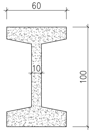
a-a kesiti
